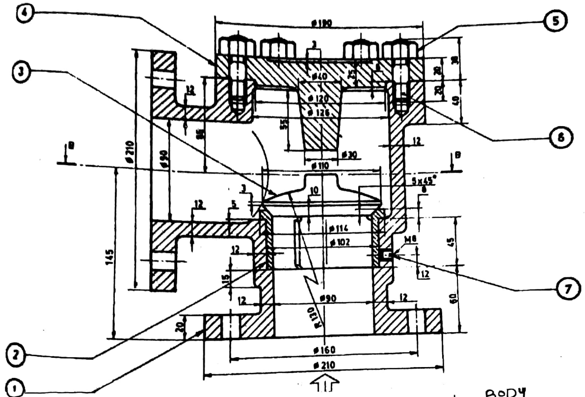
Fig. IV Non return valve .
